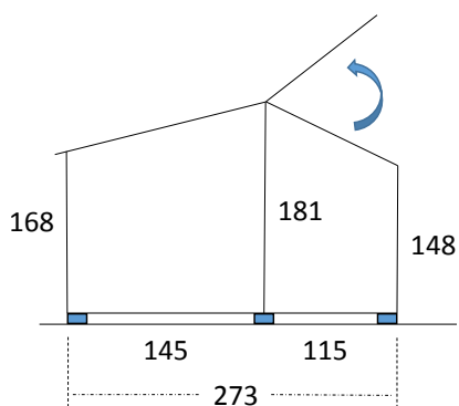
buitenafmetingen (cm) LSC150300-RGH buitenafmetingen (cm) LSC175300-RGH
