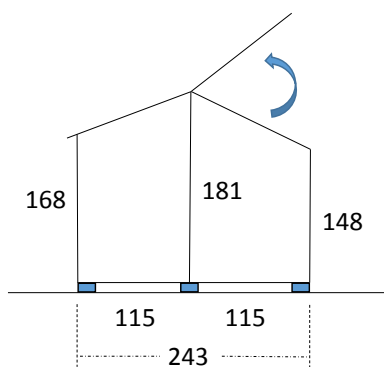
buitenafmetingen (cm) LSC150-RGH buitenafmetingen (cm) LSC175-RGH
